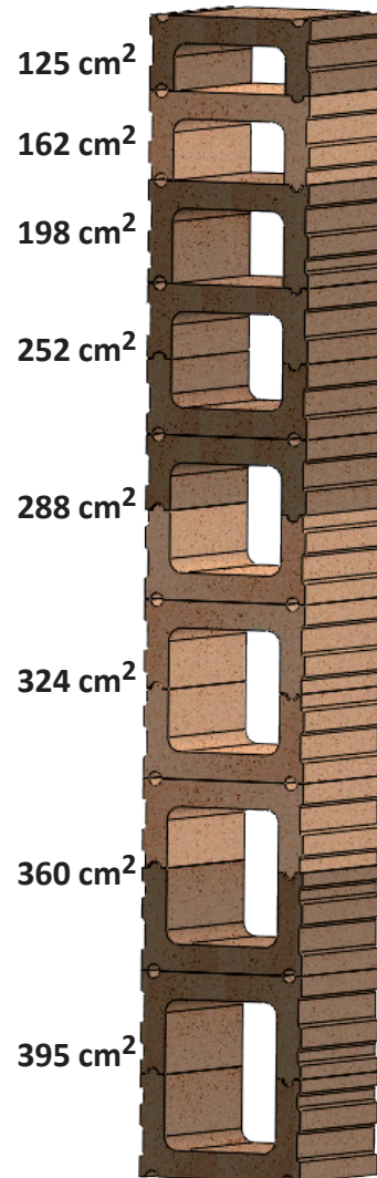
Starterset 2 Zuglänge ca. 3,5m ArtNr. 1kafSta2
